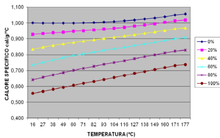
CALORE SPECIFICO DI SOLUZIONI ACQUOSE IN LIQUIDO PURO
