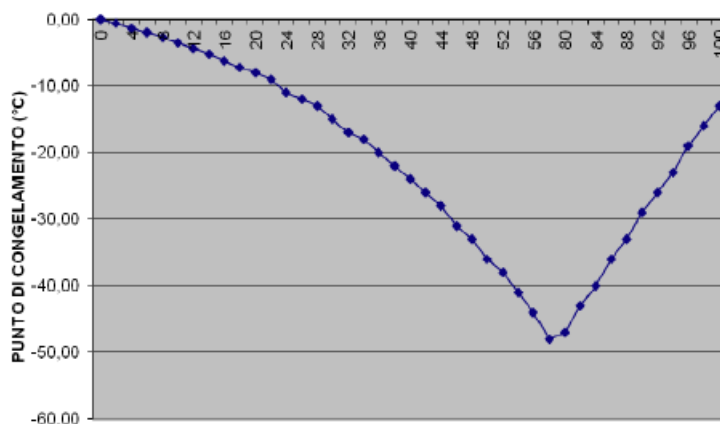
ANDAMENTO PUNTO DI CONGELAMENTO (°C)
